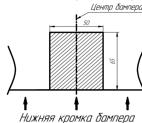
Схема 1 - Подрезка бампера
